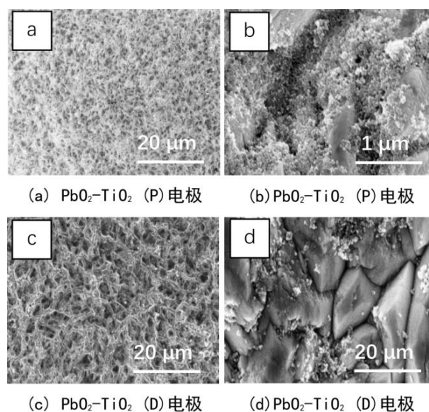
图3 \text{PbO}_2\text{-TiO}_2 (P) 和 \text{PbO}_2\text{-TiO}_2 (D) 电极的 SEM 照片
